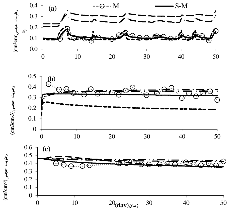
شکل ۱- شبیه‌سازی تغییرات زمانی رطوبت خاک برای اعماق 15 (a)، 45 (b) و 75 (c) سانتی‌متر. M : رطوبت اندازه‌گیری شده، S-M ، S-W(1997) ، S-W(1999) ، S-Gh\&H(Adj.) : رطوبت شبیه‌سازی شده با HYDRUS-1D به ترتیب با بکارگیری منحنی رطوبتی برازش یافته به مقادیر اندازه‌گیری شده با RETC و برآورد شده با توابع انتقالی وستن (1997) ، وستن (1999) و قربانی اصلاح شده.
